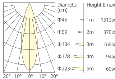
7W/24°/3000K/Ra90
