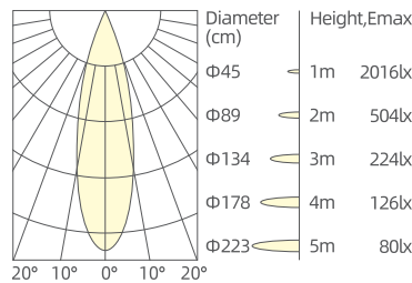
9W/24°/3000K/Ra90
