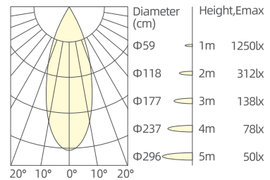
9W/36°/3000K/Ra90
