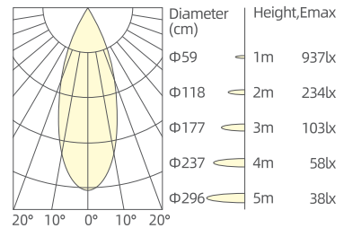
7W/36°/3000K/Ra90
