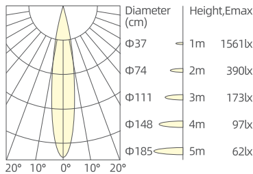
7W/15°/3000K/Ra90
