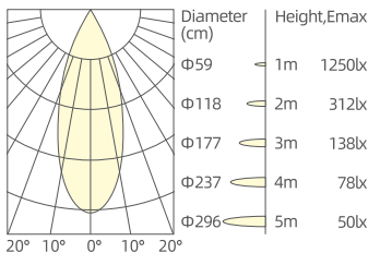
9W/36°/3000K/Ra90
