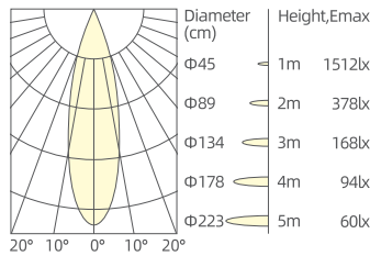
7W/24°/3000K/Ra90
