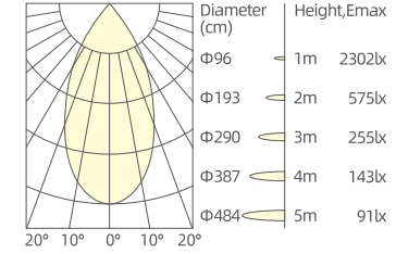
20W/50°/3000K/Ra90
