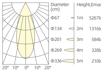
25W/36°/3000K/Ra90
