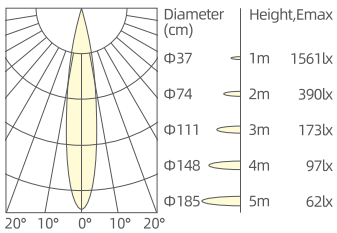
7W/15°/3000K/Ra90
