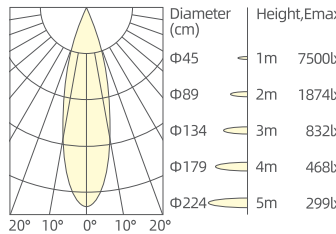
20W/24°/3000K/Ra90
