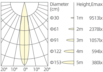
20W/15°/3000K/Ra90
