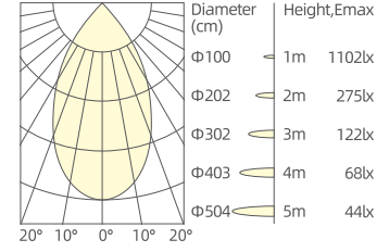
20W/50°/3000K/Ra90
