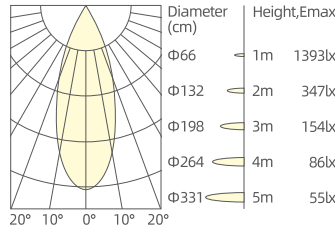
10.5W/36°/3000K/Ra90
