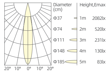
9W/24°/3000K/Ra90
