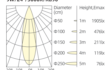
9W/24°/3000K/Ra90
