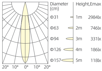
6W/15°/3000K/Ra90
