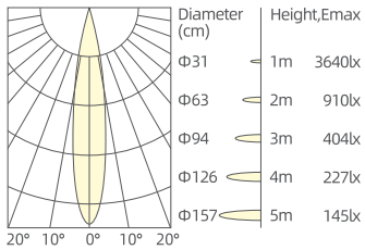
8W/15°/3000K/Ra90
