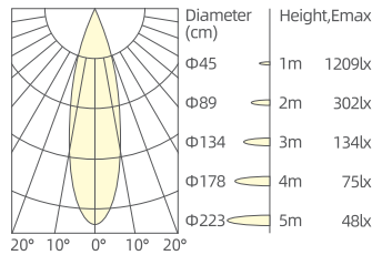
4W/24°/3000K/Ra90
