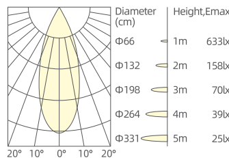
5W/36°/3000K/Ra90
