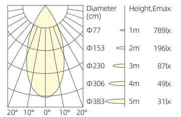
6W/50°/3000K/Ra90
