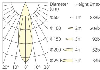
4W/24°/3000K/Ra90
