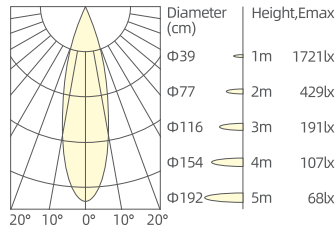
6W/24°/3000K/Ra90
