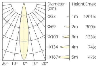
4W/15°/3000K/Ra90
