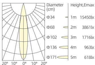
3x14W/15°/3000K/Ra90
