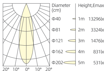
3x14W/24°/3000K/Ra90
