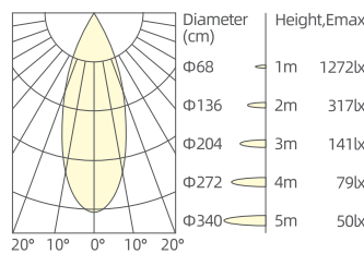
3x10W/36°/3000K/Ra90
