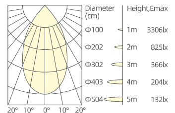
3x14W/55°/3000K/Ra90
