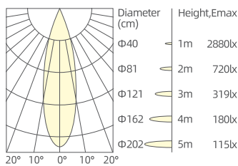
3x10W/24°/3000K/Ra90
