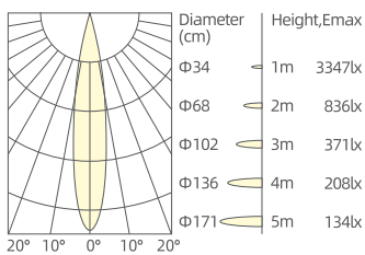
3x10W/15°/3000K/Ra90
