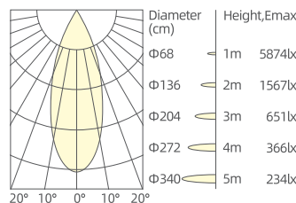
3x14W/36°/3000K/Ra90
