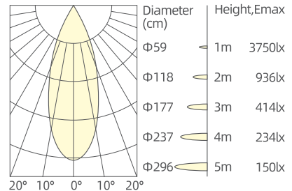
3x9W/36°/3000K/Ra90
