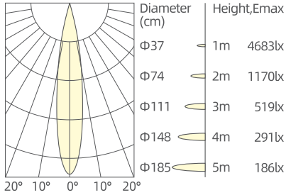
3x7W/15°/3000K/Ra90
