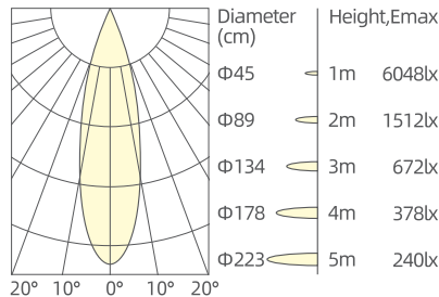
3x9W/24°/3000K/Ra90
