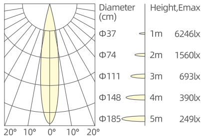
3x9W/15°/3000K/Ra90
