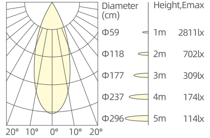
3x7W/36°/3000K/Ra90
