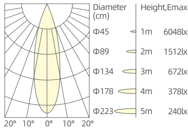
3x9W/24°/3000K/Ra90
