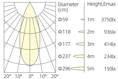
3x9W/36°/3000K/Ra90
