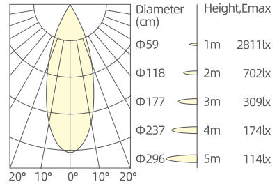
3x7W/36°/3000K/Ra90
