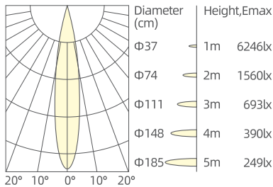
3x9W/15°/3000K/Ra90
