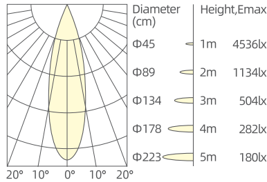
3x7W/24°/3000K/Ra90
