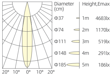
3x7W/15°/3000K/Ra90
