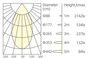
3x9W/45°/3000K/Ra90
