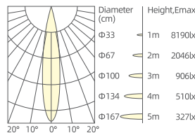
3x9W/15°/3000K/Ra90
