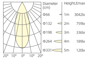
3x9W/24°/3000K/Ra90
