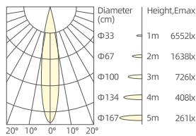
3x9W/10°/3000K/Ra90
