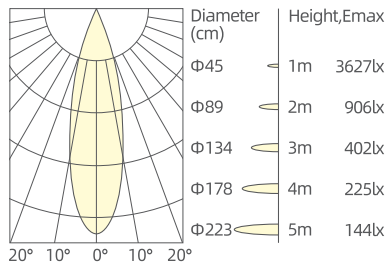
3x4W/24°/3000K/Ra90
