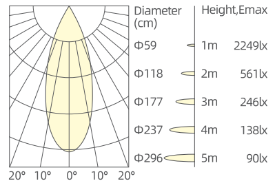
3x4W/36°/3000K/Ra90
